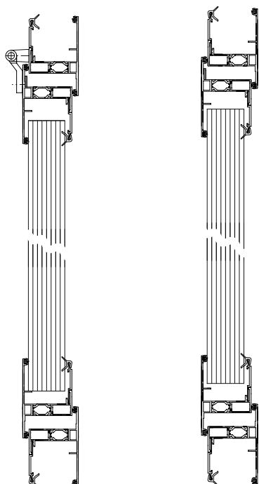
svislý řez
